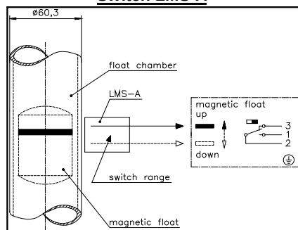
Switch LMS-A
