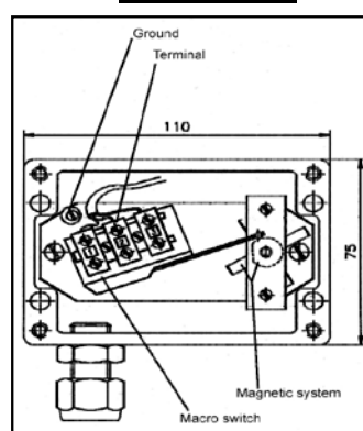
Switch MS09K
