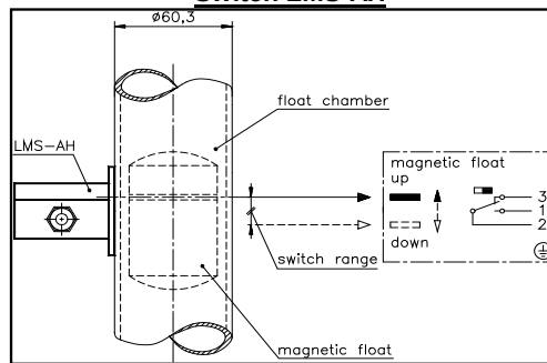
Switch LMS-AH
