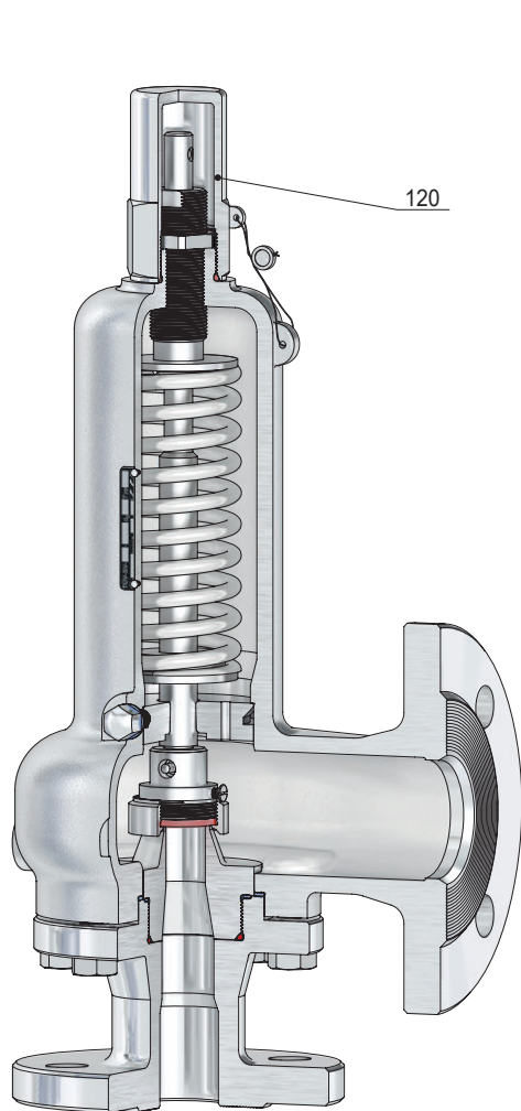
BG III Kopf C
